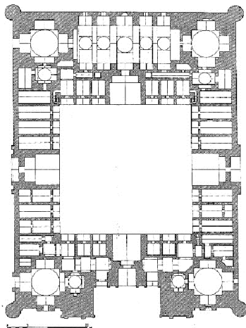
План 6: Медресе Улуу Бей Самарканда
