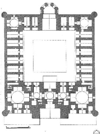
План 8: Медресе Улуу Бей Бухары
