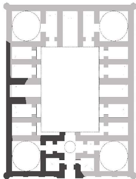
План-1а: Наше предложение реституции после данных раскопок и публикаций Немцевой-Шваба
