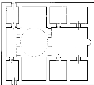
План 5: Медресе Гюмюштекина в Босре(1136)(по Созену)
