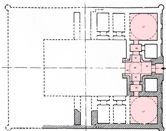
План 2: Входная часть медресе и пространства связанные с этой частью
