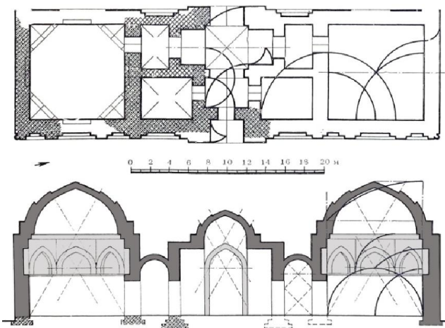
Рисунок-3: План восточного фасада(вход) и сечение, подготовленные после раскопок медресе(по Немцевой-Швабу)
