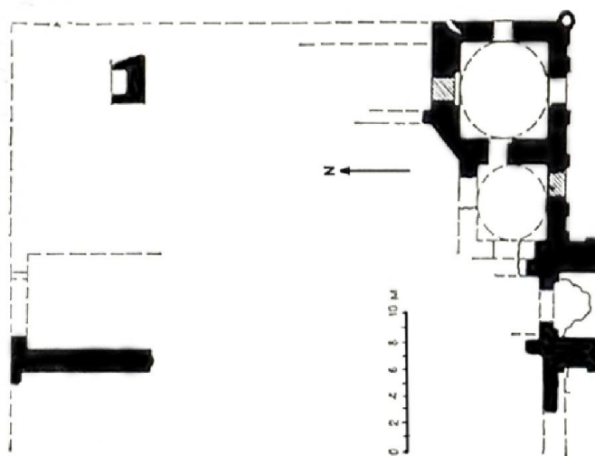
План 4а: Медресе Шахи Мешхеда в Афганистане (12век) (по Немцевой-Швабу)
