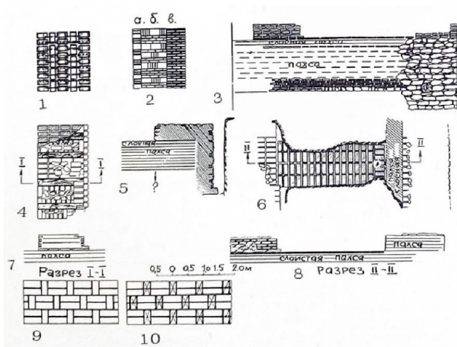
Рисунок 5: Фрагменты основных и стенных материалов, а также техники использования, обнаруженные во время раскопок (по Немцевой-Швабу)
