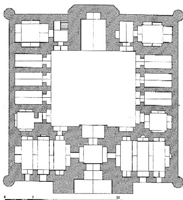
План 7: Медресе Улуу Бей Гучдевана
