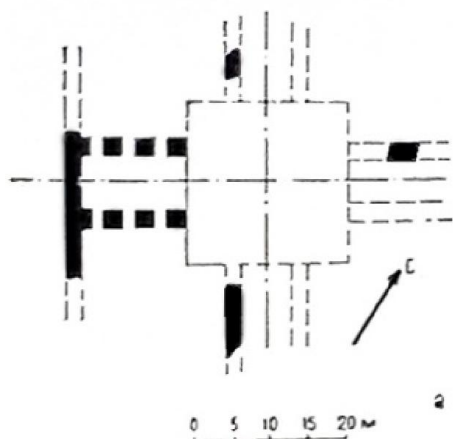
План 3: Медресе Харджита в Хорасане (1084) (по Немцевой-Швабу)
